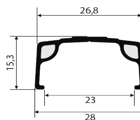
NI-381 0,219 kg/m
