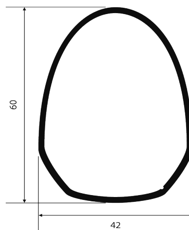
NI-248 0,695 kg/m
