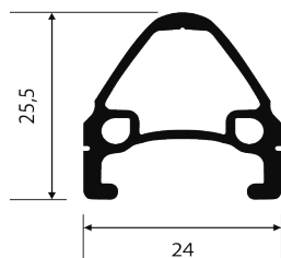
NI-377 0,329 kg/m
