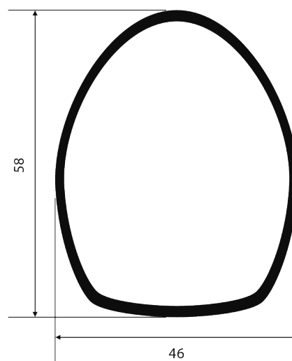
XKS-02 0,747 kg/m
