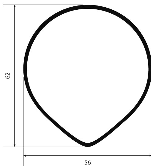
XKS-03 0,762 kg/m
