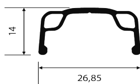
NI-306 0,202 kg/m
