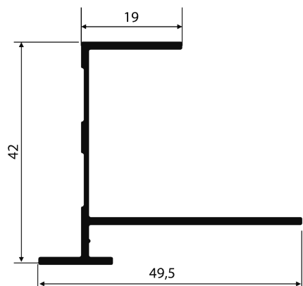
NI-366 0,428 kg/m
