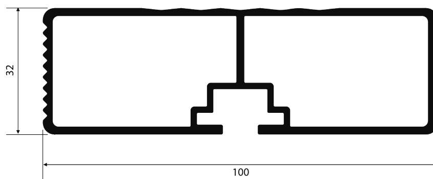
NI-537 1,353 kg/m
