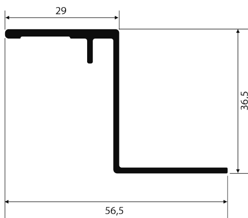
NI-365 0,445 kg/m
