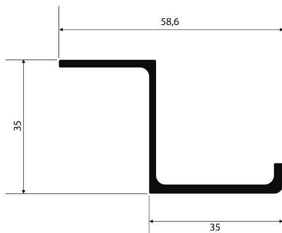
NI-031 0,557 kg/m
