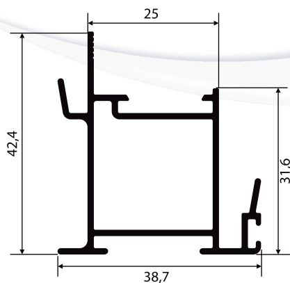
SU-042 0,563 Kg/m
