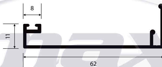
NI-117 0,327 Kg/m
