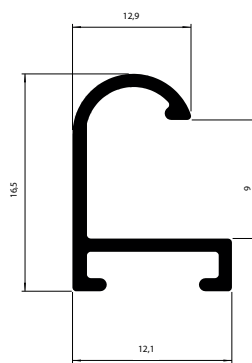
NI-541 0,115 Kg/m
