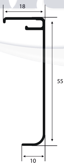
BX-157 0,220 Kg/m
