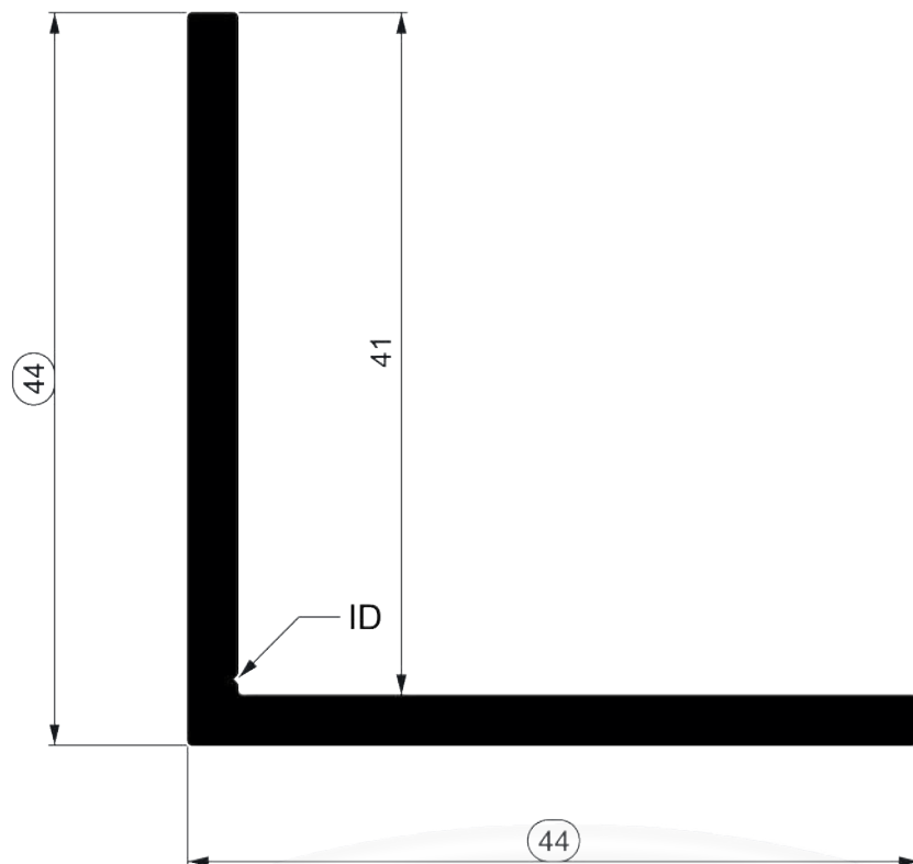
NI-2461 0,691 Kg/m
