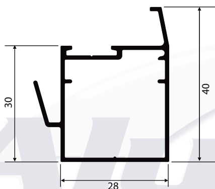
NI-562 0,453 Kg/m
