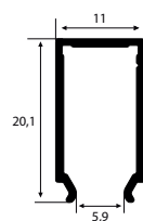
NI-1663 0,134 Kg/m
