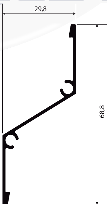
VZ-060 0,369 Kg/m
