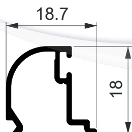
LG-026 0,155 Kg/m
