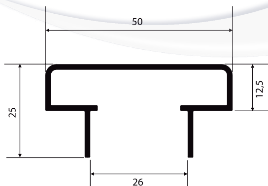
CG-731 0,487 Kg/m
