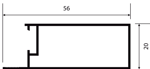
MP-336 0,424 Kg/m
