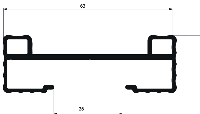
NI-1209 0,680 Kg/m
