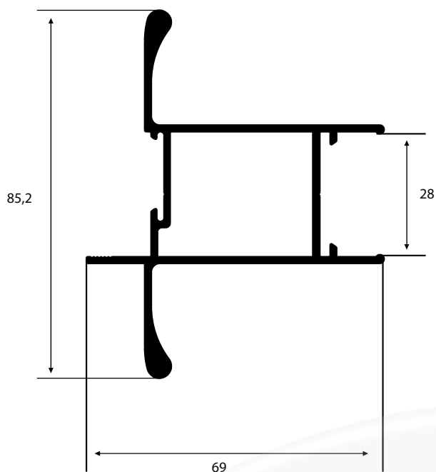
LG-201 1,181 Kg/m
