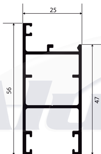
A-048 0,645 Kg/m
