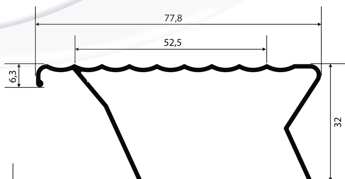
NI-1137 0,504 Kg/m
