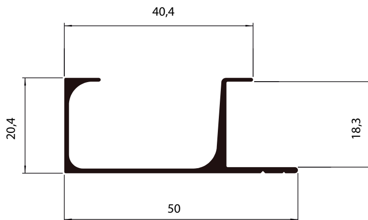
NI-4058 0,341 Kg/m
