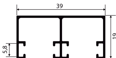
NI-971 0,344 Kg/m
