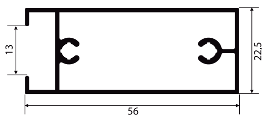
NI-012 0,593 Kg/m
