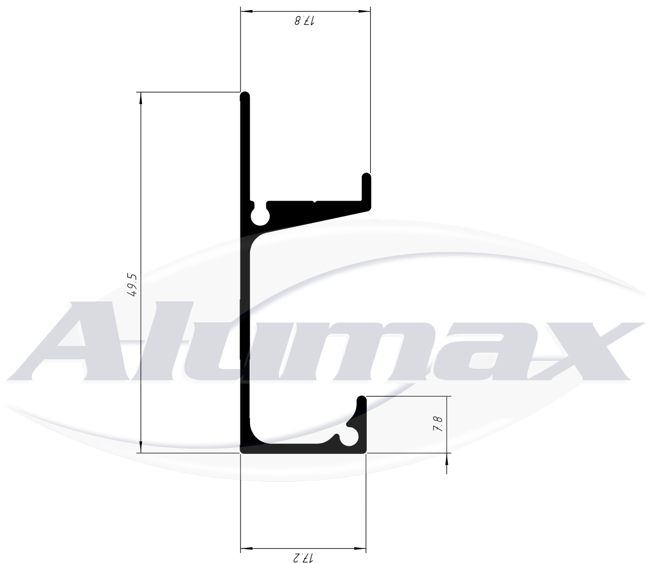
NI-4065 0,372 Kg/m
