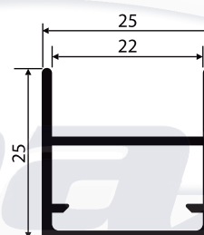
A-056 0,373 Kg/m
