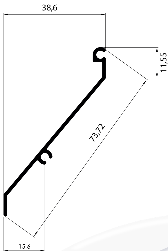
NI-1308 0,277 Kg/m
