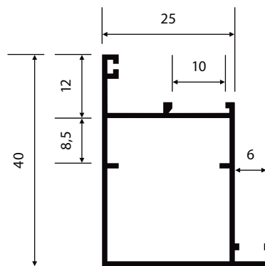
P-151 0,496 Kg/m
