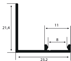
NI-1662 0,134 Kg/m
