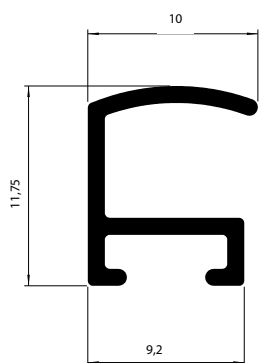
NI-539 0,090 Kg/m
