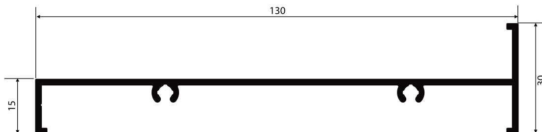
Y-350 0,950 Kg/m
