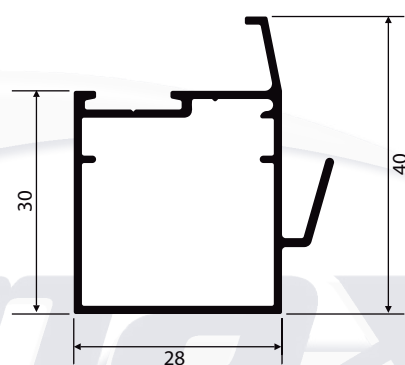
NI-563 0,455 Kg/m
