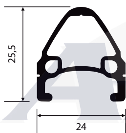
NI-377 0,329 Kg/m
