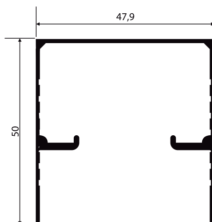
U-655 0,601 Kg/m
