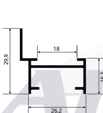
SU-071 0,283 Kg/m
