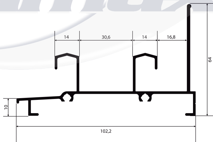
NI-522 1,206 Kg/m
