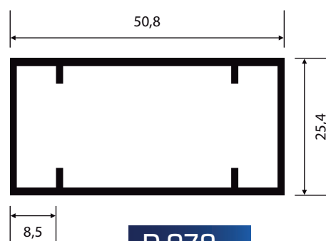
D-079 0,562 Kg/m
