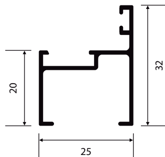
25-311 0,287 Kg/m
