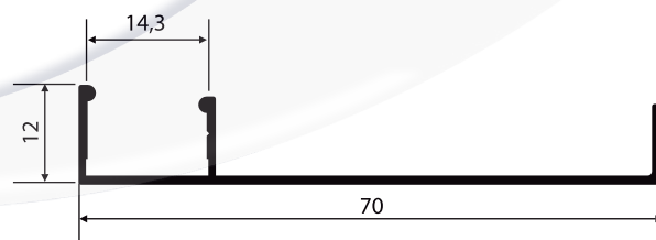
NI-944 0,301 Kg/m
