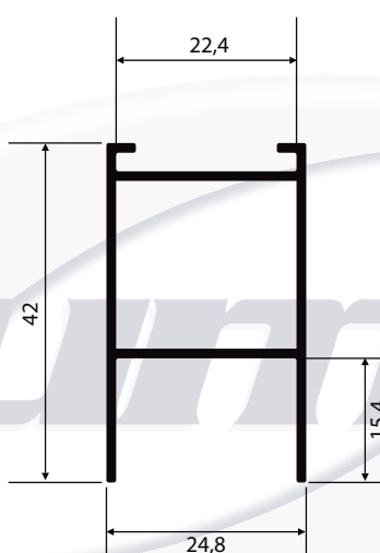
SU-072 0,435 Kg/m
