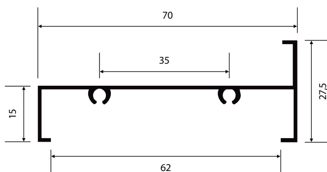
Z-175 0,533 Kg/m
