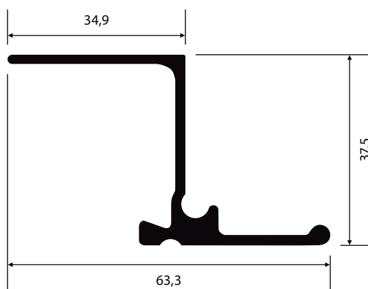
NI-207 0,706 Kg/m
