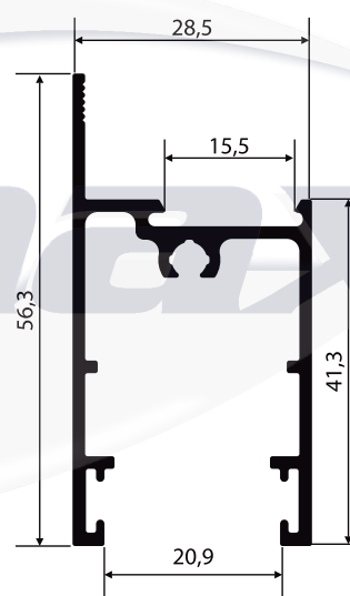
NI-507 0,655 Kg/m
