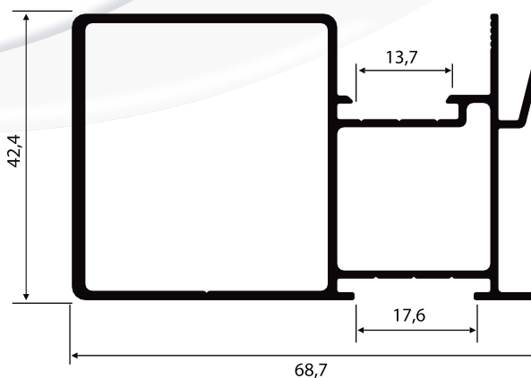
SU-047 1,041 Kg/m
