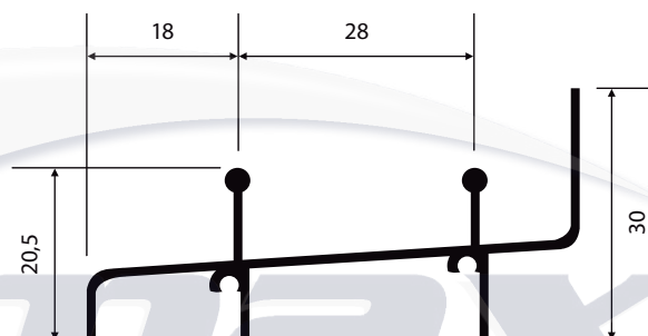
MP-370 0,565 Kg/m
