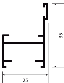
SU-079 0,332 Kg/m
