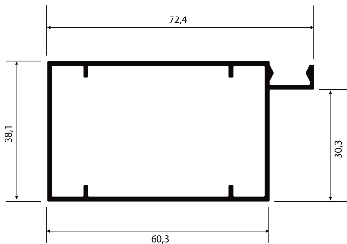
NI-405 0,795 Kg/m
