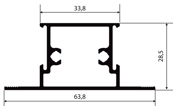
NI-516 0,742 Kg/m
