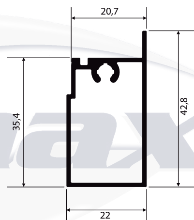
SU-073 0,457 Kg/m
