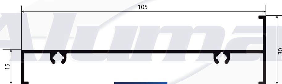
Y-260 0,658 Kg/m
