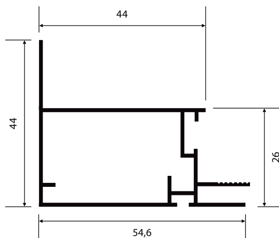
MP-069 0,602 Kg/m
