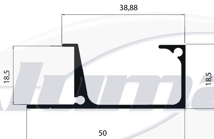
NI-4064 0,422 Kg/m
