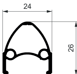
NI-2267 0,296 Kg/m
