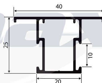
NI-762 0,376 Kg/m
