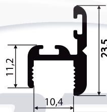
Y-343A 0,279 Kg/m
