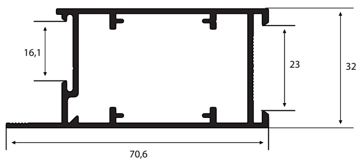
LG-043 0,834 Kg/m
