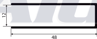
NI-841 0,350 Kg/m
