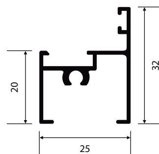
25-312 0,321 Kg/m
