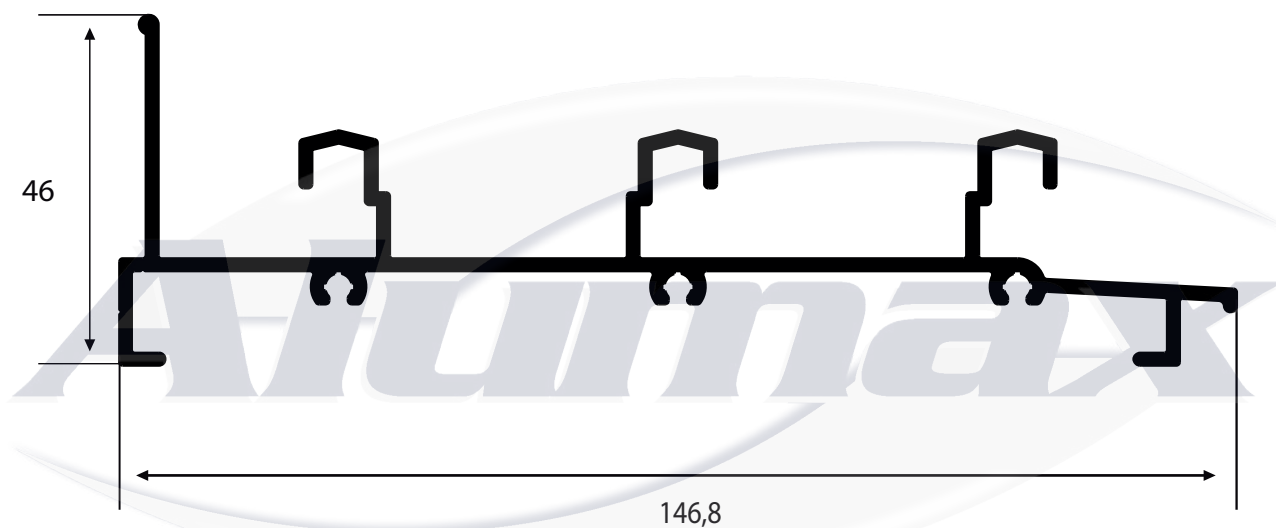
NI-1466 1,446 Kg/m
