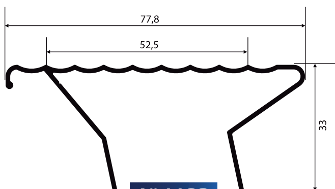
NI-1138 0,532 Kg/m
