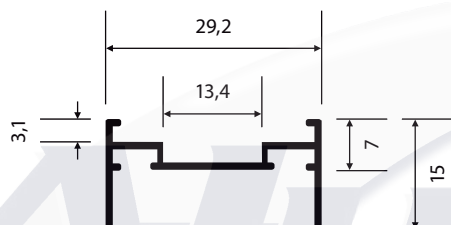
I-105 0,220 Kg/m
