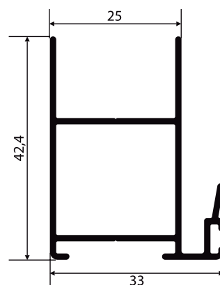
SU-070 0,518 Kg/m
