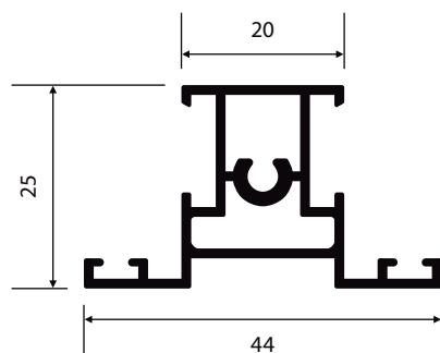
MM-376 0,521 Kg/m
