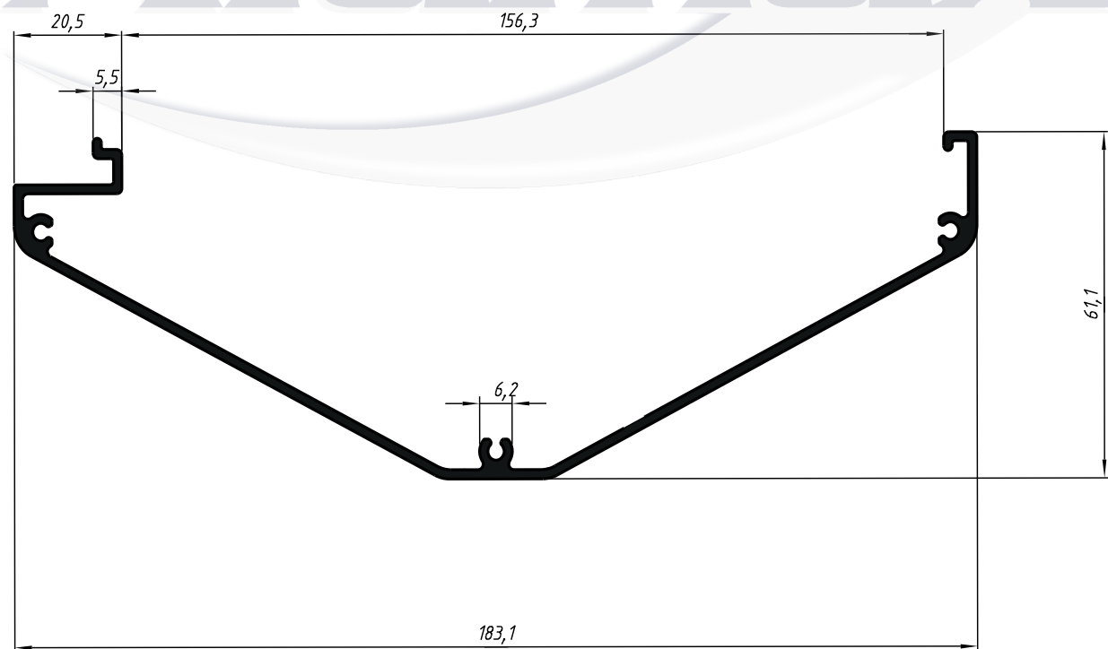
MN-008 1,325 Kg/m
