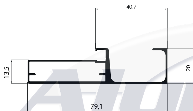
NI-7035 0,612 Kg/m
