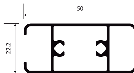
SU-188 0,591 Kg/m
