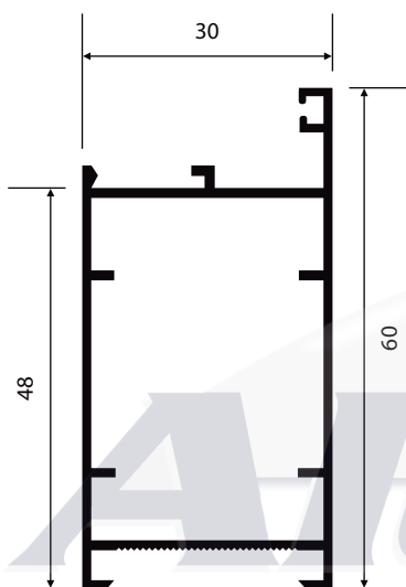
P-270 0,793 Kg/m
