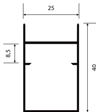
A-055 0,434 Kg/m
