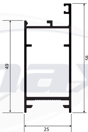
P-414 0,611 Kg/m
