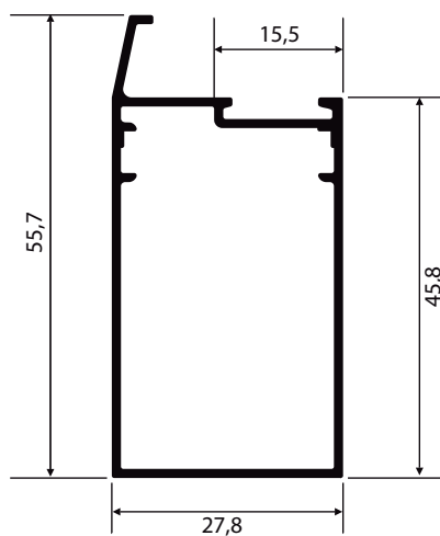
NI-565 0,502 Kg/m
