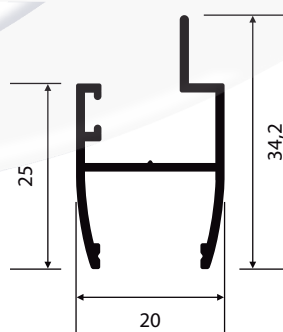
LE-1628 0,295 Kg/m
