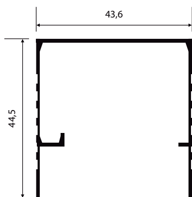
NI-150 0,421 Kg/m
