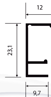
ME-092 0,173 Kg/m
