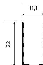
U-556 0,142 Kg/m
