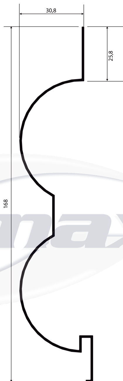
LB-070 0,763 Kg/m
