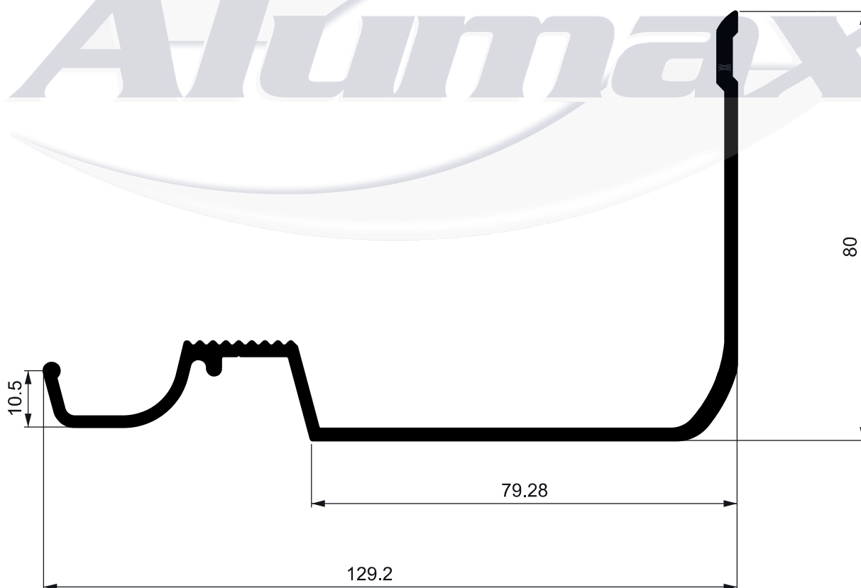
NI-2461 0,691 Kg/m
