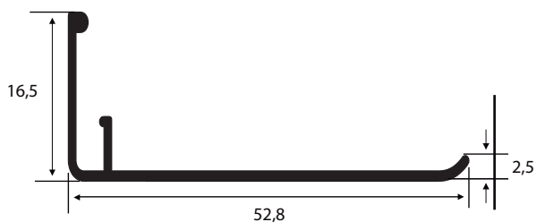
NI-801 0,207 Kg/m
