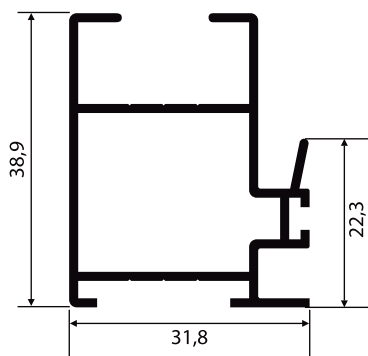
SU-056 0,541 Kg/m
