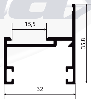
LG-083 0,411 Kg/m
