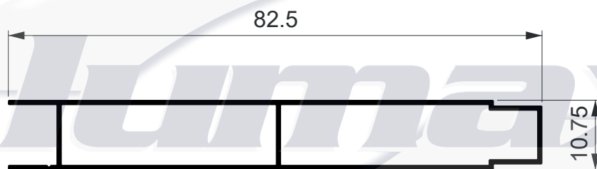
NI-2271 1,465 Kg/m
