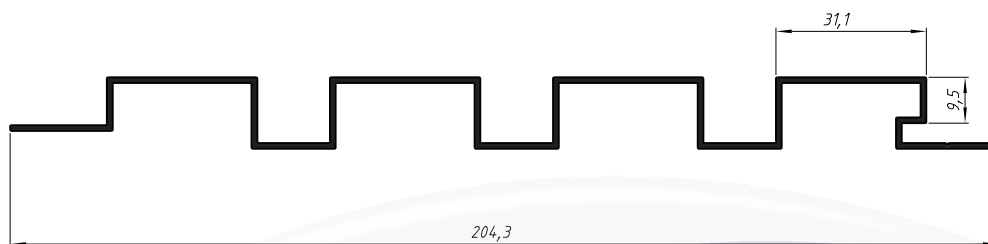
NI-2078 1,046 Kg/m
