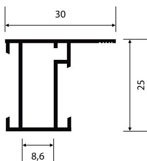
SU-080 0,355 Kg/m
