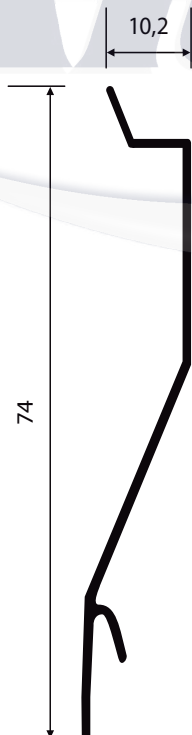
VZ-051 0,269 Kg/m
