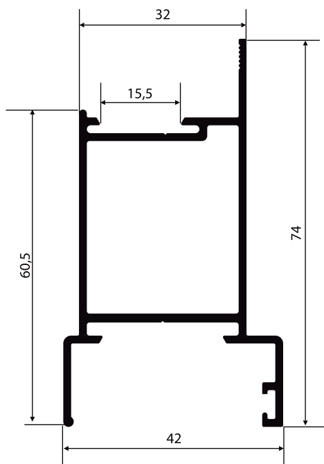
NI-515 0,920 Kg/m
