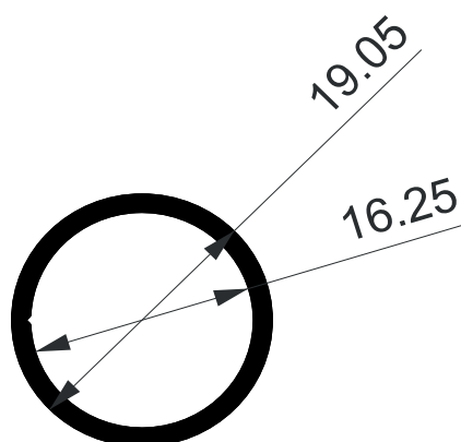
NI-2265 0,210 Kg/m
