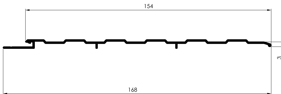
Y-429L 0,526 Kg/m
