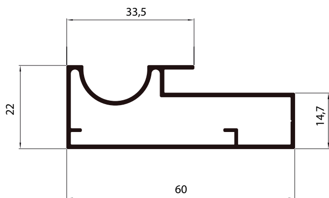
NI-7014 0,509 Kg/m
