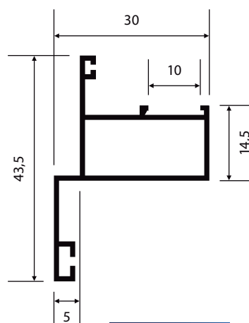
P-146 0,466 Kg/m
