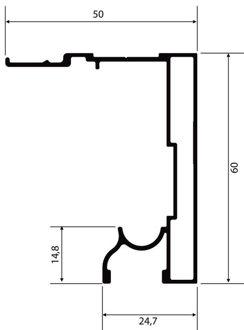
NI-446 0,654 Kg/m
