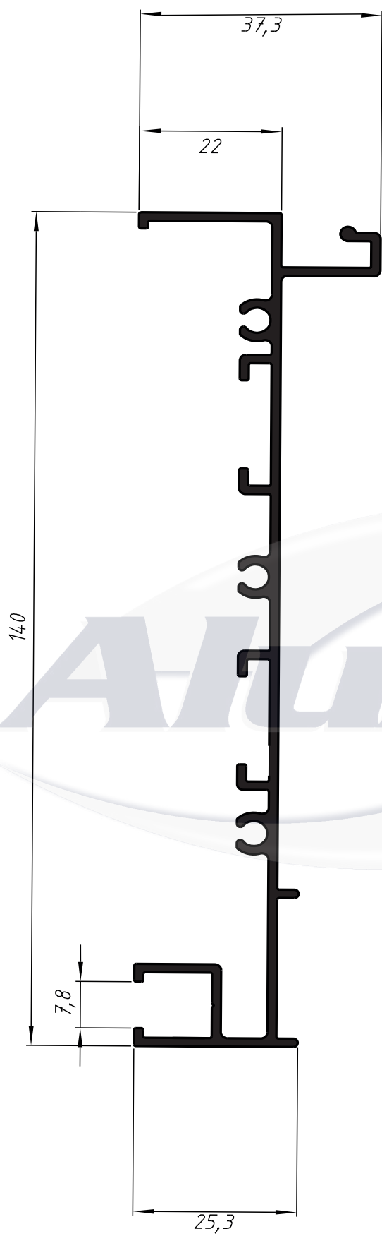
MN-001 1,179 Kg/m
