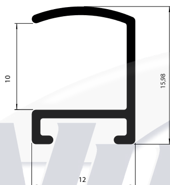
NI-540 0,115 Kg/m
