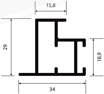
NI-162 0,483 Kg/m
