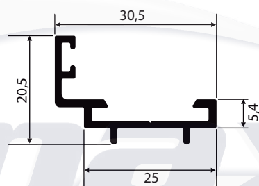
L-715 0,255 Kg/m
