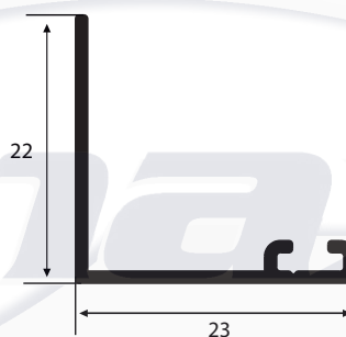
NI-1315 0,137 Kg/m
