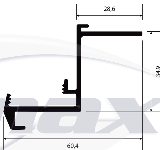
NI-064 0,733 Kg/m
