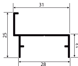
NI-758 0,215 Kg/m
