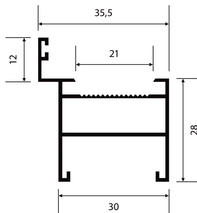
P-273 0,563 Kg/m
