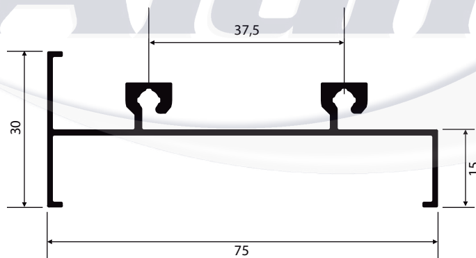
NI-569 0,613 Kg/m
