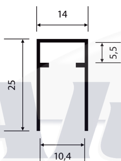
U-1056 0,183 Kg/m
