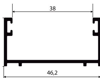
NI-509 0,436 Kg/m
