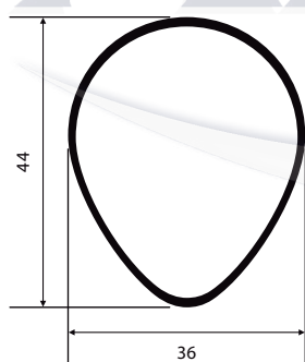
XKS-01 0,530 Kg/m
