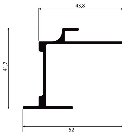
NI-486 0,539 Kg/m
