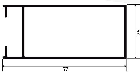
NI-011 0,503 Kg/m
