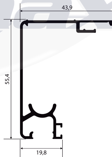
NI-939 0,579 Kg/m
