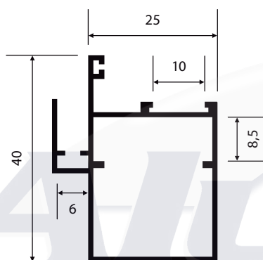
P-152 0,523 Kg/m
