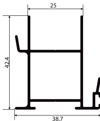
SU-069 0,576 Kg/m
