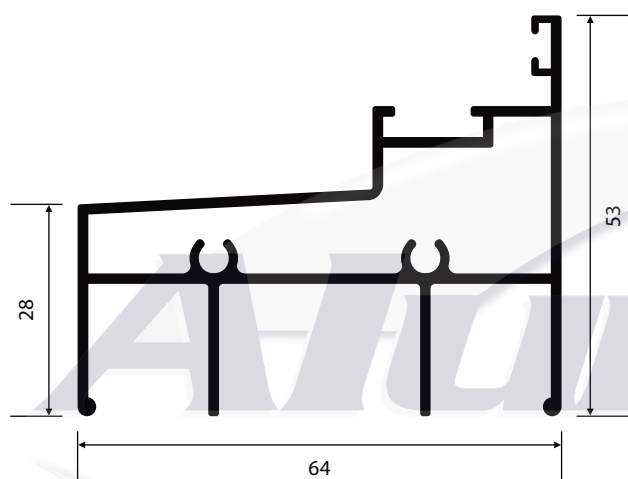
MP-361 1,074 Kg/m
