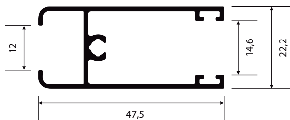
SU-186 0,507 Kg/m
