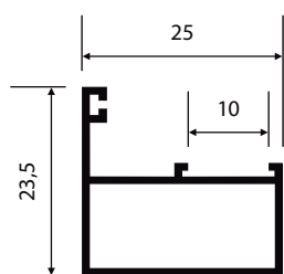
P-147 0,351 Kg/m
