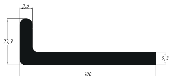
NI-2155 3,115 Kg/m
