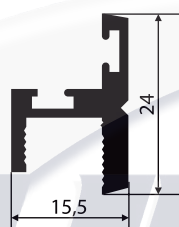
Y-343 0,314 Kg/m
