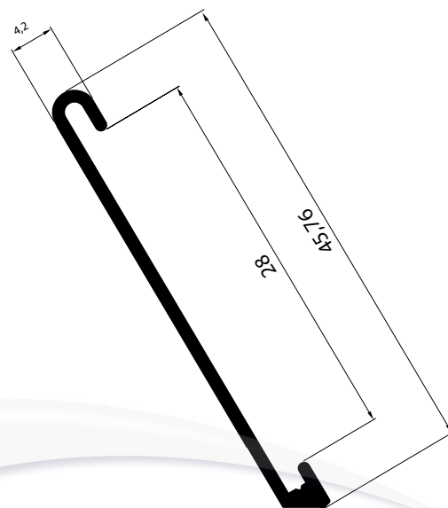
NI-1372 0,185 Kg/m
