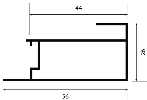
MP-070 0,497 Kg/m
