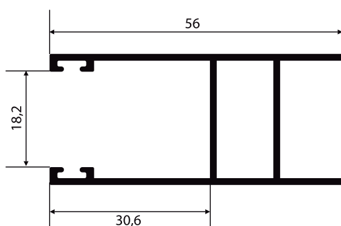
A-195 0,599 Kg/m
