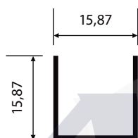
U-2020 0,158 Kg/m
