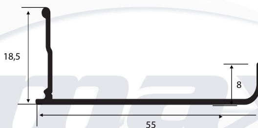
NI-1370 0,218 Kg/m
