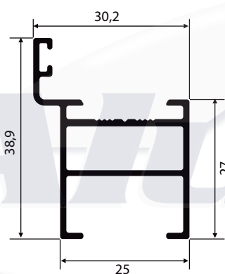
P-412A 0,439 Kg/m
