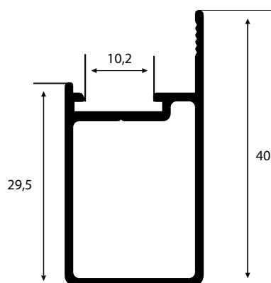
MP-300MA 0,307 Kg/m
